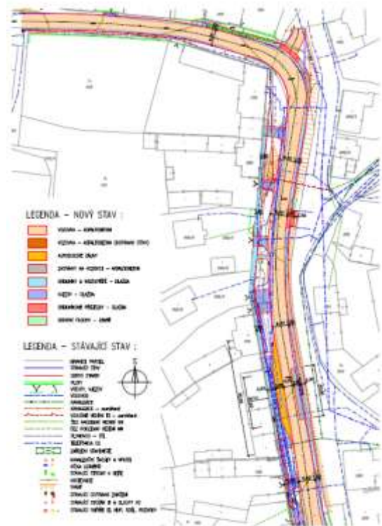
Projektová dokumentace na řešení křižovatky v Záluží, včetně autobusových zastávek a chodníků
